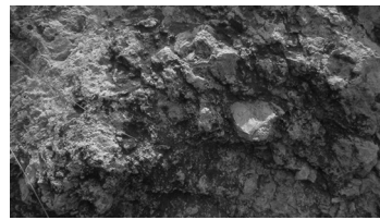
unfamiliar.JPG
