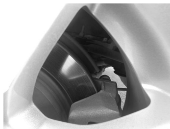
Permanent.JPG
